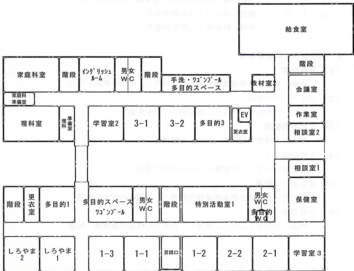
新校舎 1階
